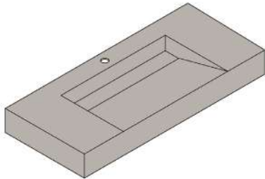
S/P Lavabo integrado 119 seno rampa C Dim. 455P x 1190L x 120H mm | CC950
