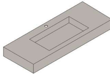
S/P Lavabo integrado 119 seno recto C Dim. 455P x 1190L x 120H mm | CC950
